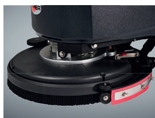
O bocal pode ser colocado e retirado sem necessidade de ferramentas, simplificando a manutenção
